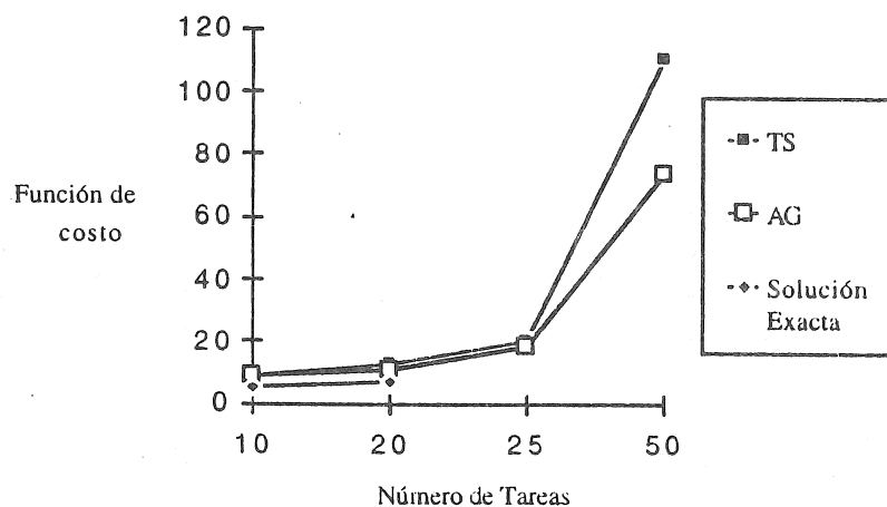
Figura 3. Optimización de la Función de Costo F_5
