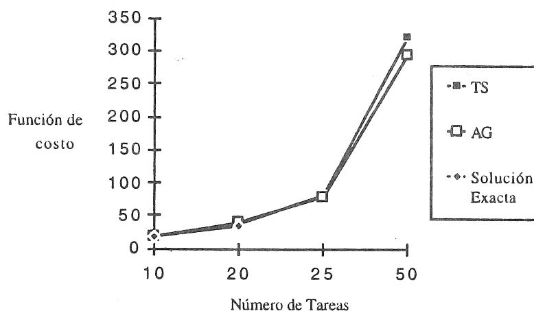
Figura 2. Optimización de la función de costo F_4
