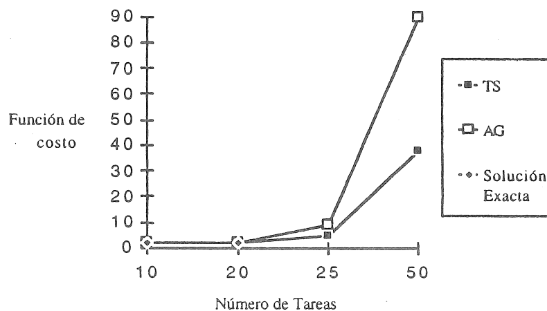
Figura 1 Optimización de la Función de Costo F_1
